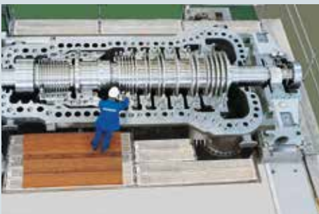
SST-800 型 (功率可达150MW)
